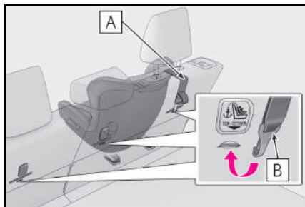
A 상부 스트랩
